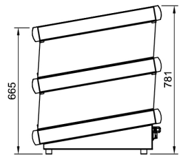
End Elevation
