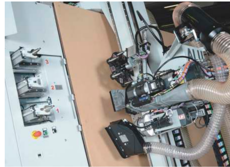
Tool changer
