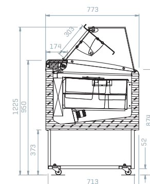
VETRO DRITTO / STRAIGHT GLASS GERADE SCHEIBE / VITRE DROITE
