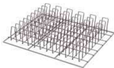
GP69 GRILL RIBS GN 2/1 AISI304 9PCS GRILLE À CÔTELETTES GN 2/1 AISI304 9 PCS ASADOR GASTRONOMICO PARA RIBS 2/1 AISI304 9 PIEZAS ПРОТИВЕНЬ ДЛЯ РЕБРЫШЕК (9 ШТ.) GN 2/1 AISI 304
