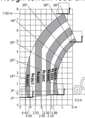
Rough terrain load chart (EN 1459 B) Metric
