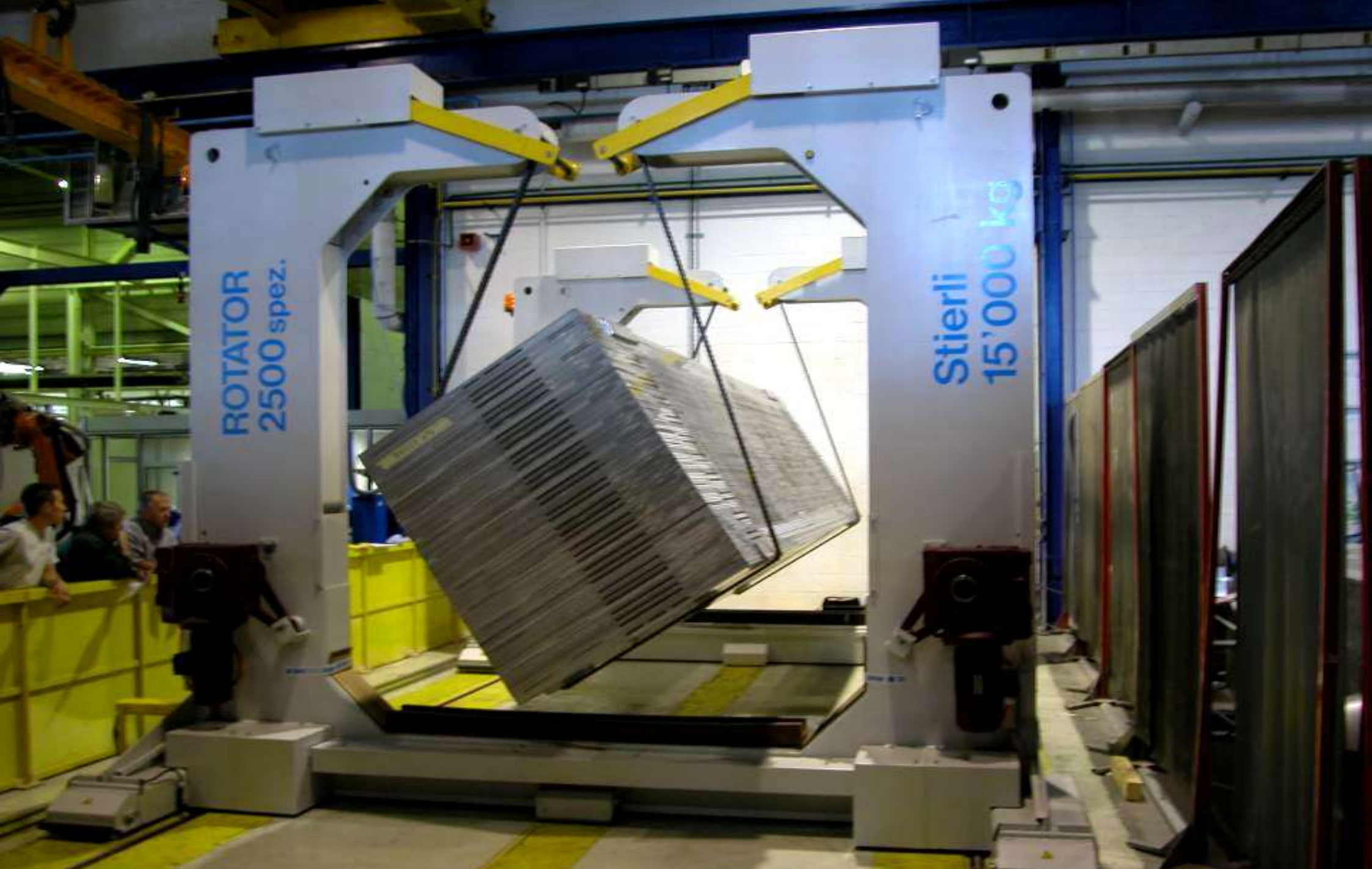
STIERLI ROTATOR
