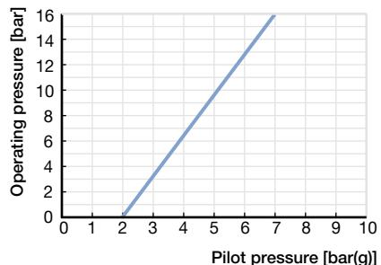
Actuator size Ø: 100(G)
