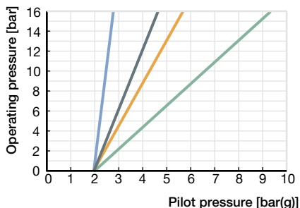
Actuator size Ø: 63(E)
