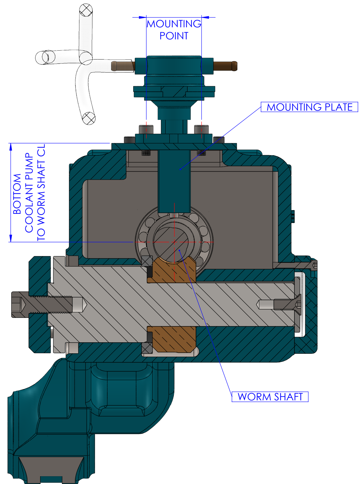
SECTION A-A
