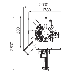
급대식 1열 자동포장기 Simplex model
