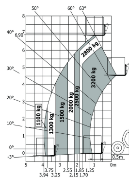
Rough terrain load chart (EN 1459 B) Metric
