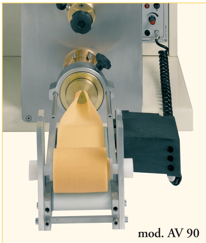
Avvolgisfoglia - Dough roller - Enrouleur d'abaisse - Teigrolle
