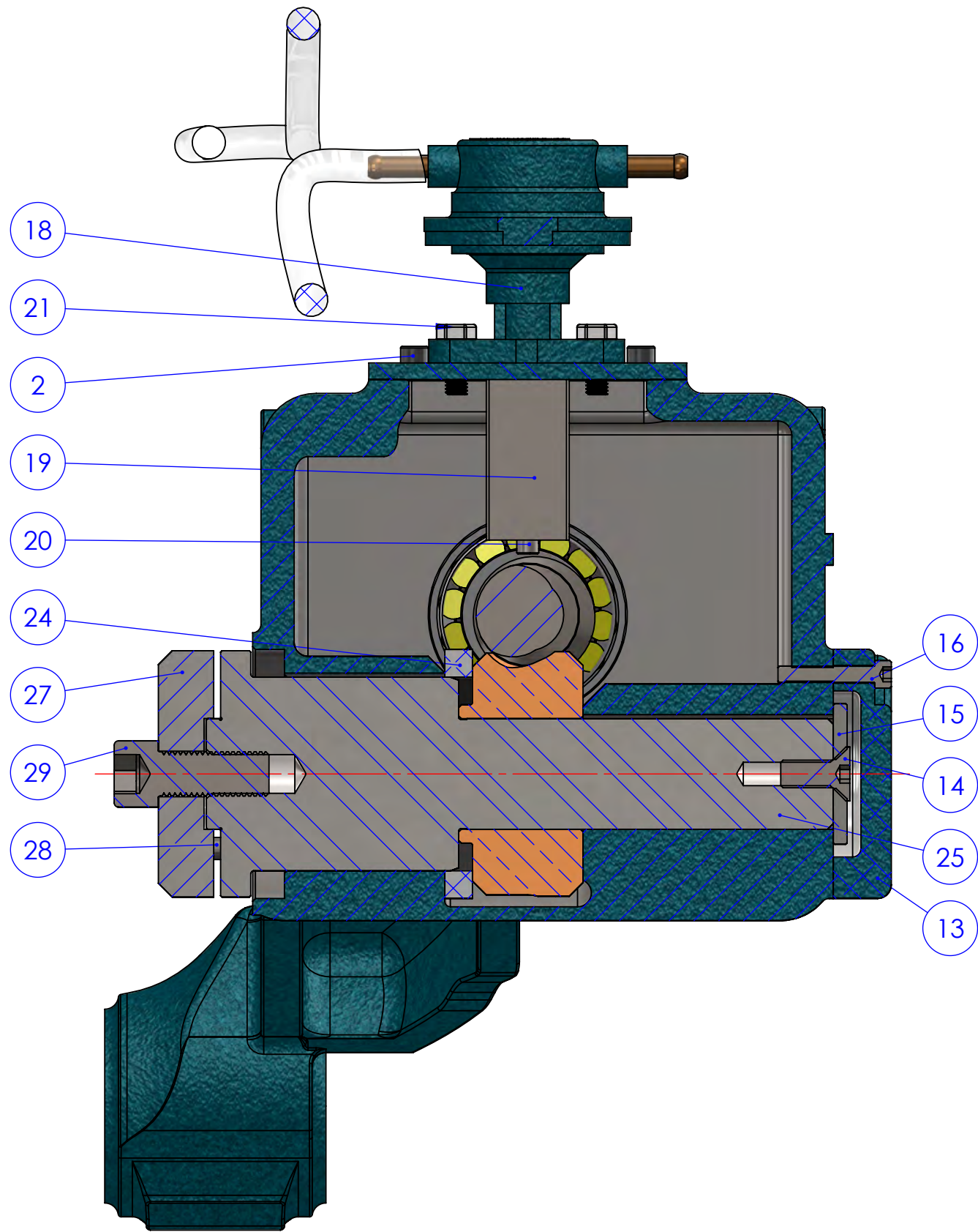
SECTION A-A
