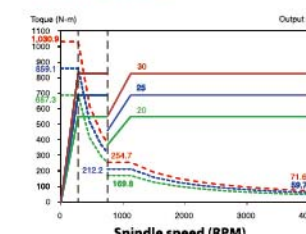
QAN260L*8000RPM
