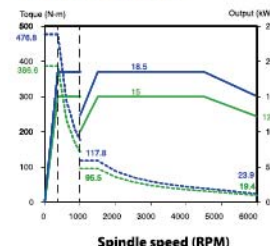
SJ-V18.5-01ZT*8000
