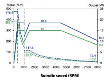
SJ-V18.5-01ZT*8000
