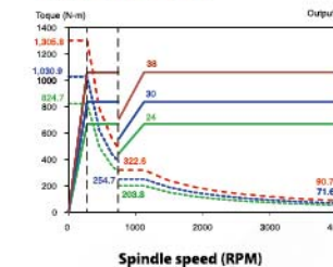
QAN260U*8000RPM
