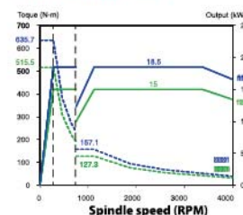
SJ-V18.5-01ZT*8000
