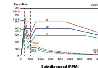
QAN260U*8000RPM
