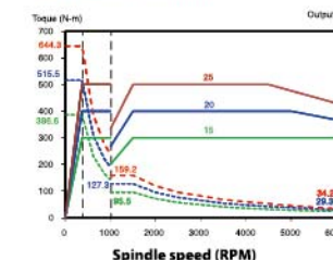
QAN260U*8000RPM
