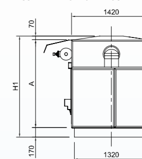
ESECUZIONE EKO...B0 SENZA ASPIRATORE ASSEMBLY EKO...B0 WITHOUT ELECTRIC FAN
