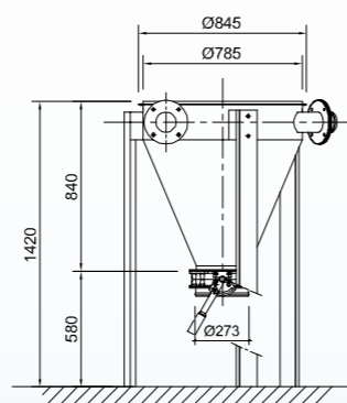
TRAMOGGIA DI RACCOLTA POLVERI DUST COLLECTOR
