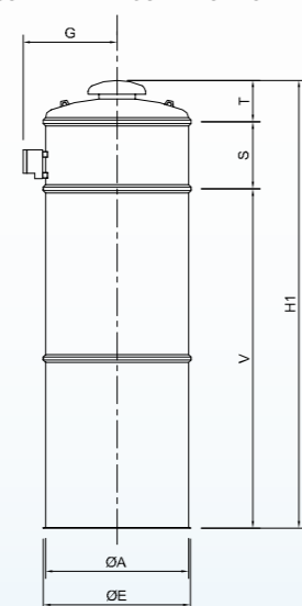
ESECUZIONE SENZA ASPIRATORE ASSEMBLY WITHOUT ELECTRIC FAN
