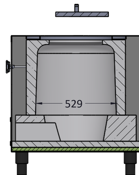
SECTION B-B SCALE 1 : 12
