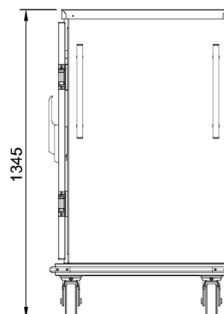
End Elevation
