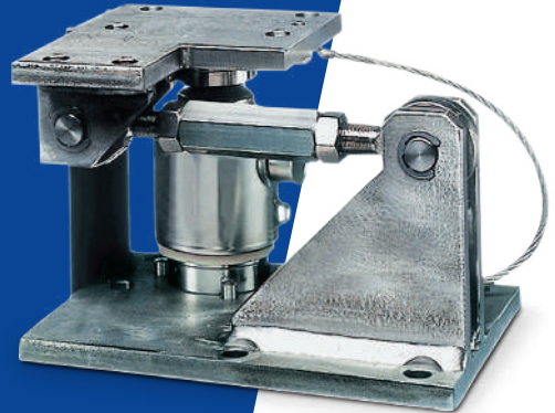
Mini FlexLock PR 6143
