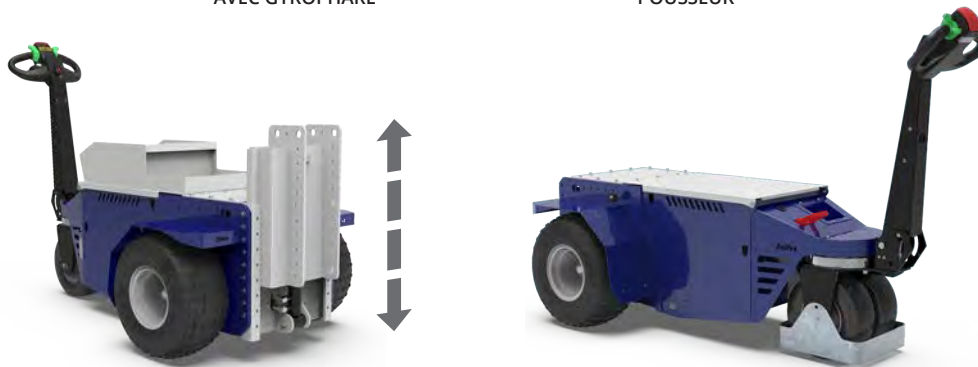
CROCHET HYDRAULIQUES POUR LE LEVAGE
