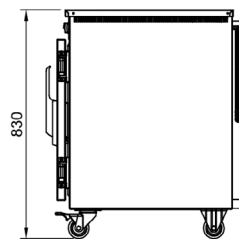
End Elevation
