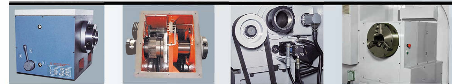
■ Headstock manual speed shifting 主軸箱手動變速 ■ Headstock / 主軸箱 ■ Headstock hyd. auto. speed shifting 主軸箱油壓自動變速 ■ Rear spindle support chuck 主軸後端支撐夾頭
