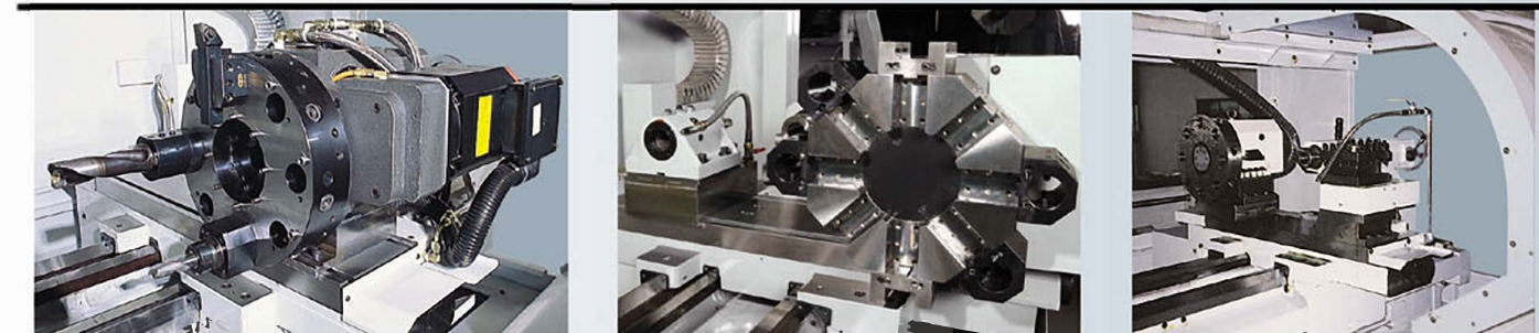
■ Driven tool system / 動力刀塔 ■ V8 turret with drill tool holder V8刀塔+鉗孔刀座 ■ Twin turret / 雙刀塔
